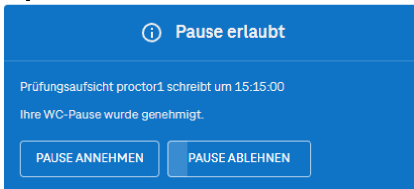
Abbildung 9: Pausenanfrage genehmigt
